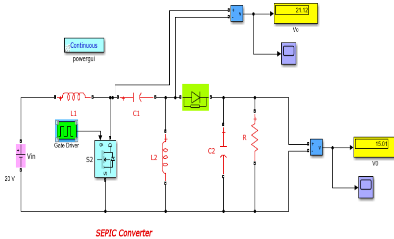
Şekil 7. Sepic çevicinin Matlab/Simulink eşdeğeri
