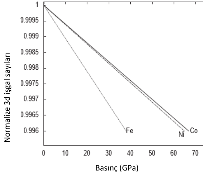
Şekil 2. Ağır geçiř metalleri için normalize 3d elektron sayısının basınçla deęiřimi
