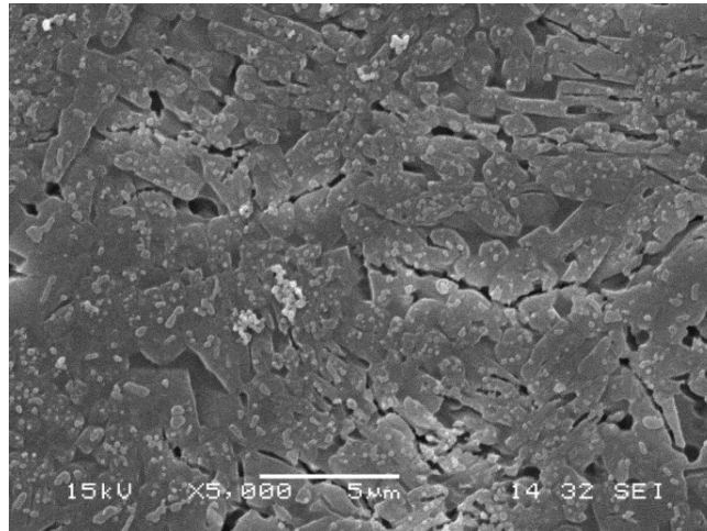
Şekil 2.2. 1350 °C’de 60 dk süre ile sinterlenmiş katkısız numunenin SEM mikrofrafı
