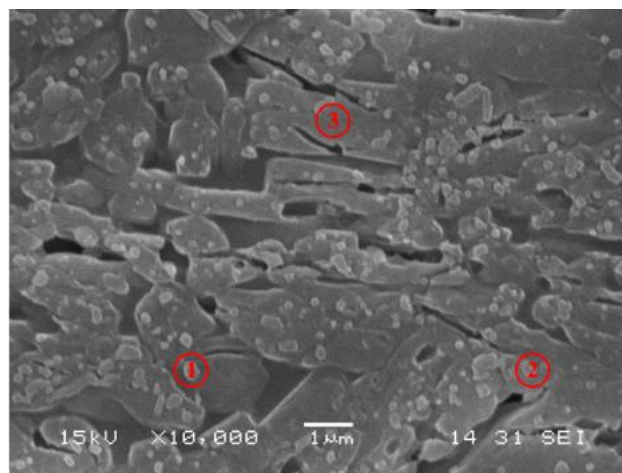
Şekil 2.2. 1350 °C’de 60 dk süre ile sinterlenmiş katkısız numunenin SEM mikrofrafı
